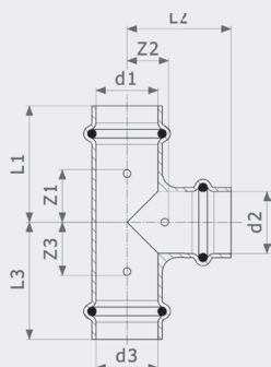
Тройник Profipress G - медь Модель 2618
