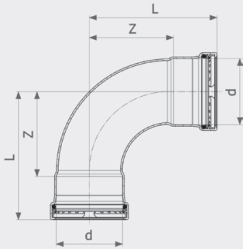
Отвод 90° Profipress G XL - медь Модель 2616XL
