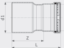
Редукционная вставка Profipress G XL - медь Модель 2615.1XL
