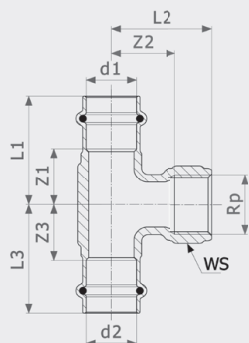
Тройник Profipress G - бронза Модель 2617.2
