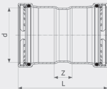
Муфта Profipress G XL - медь Модель 2615XL
