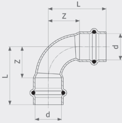
Отвод 90° Profipress G - медь Модель 2616
