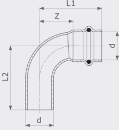
Отвод 90° Profipress G - медь Модель 2616.1
