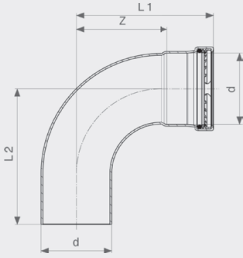
Отвод 90° Profipress G XL - медь Модель 2616.1XL
