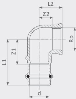
Угольник переходной 90° Profipress G - бронза Модель 2614.2
